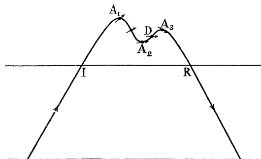
FIG. 14. A group-ray.
