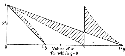
FIG. 17. The zeros of q , y < 1 .
