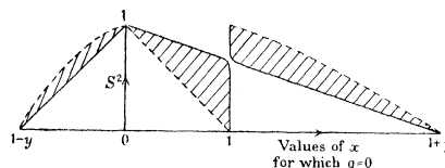
FIG. 18. The zeros of q , y > 1 .
